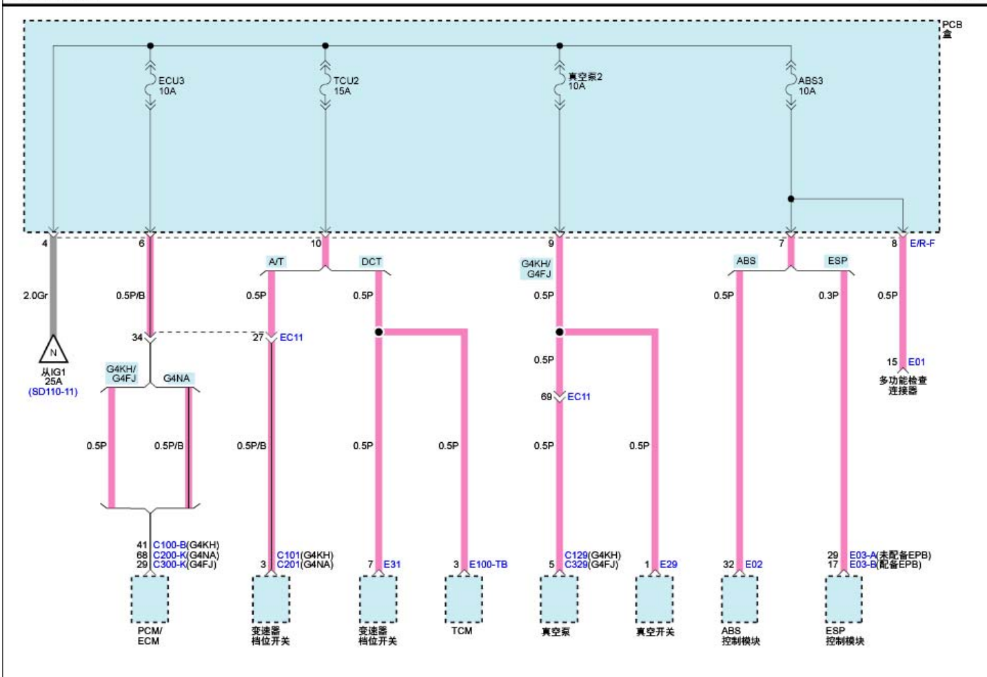
电源分布(5)
